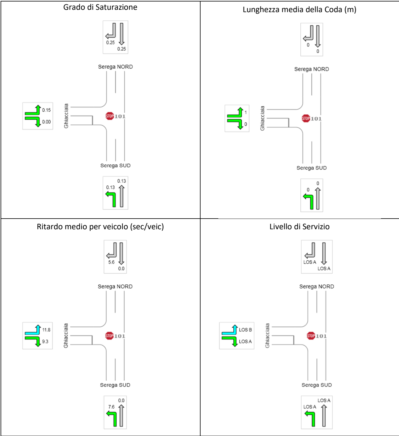
Figura 8-6: Nodo N02 – via Serega (SP 18) – via Ghiacciaia Risultati delle verifiche di capacità - Ora di Punta 17.30-18.30 – SdF
