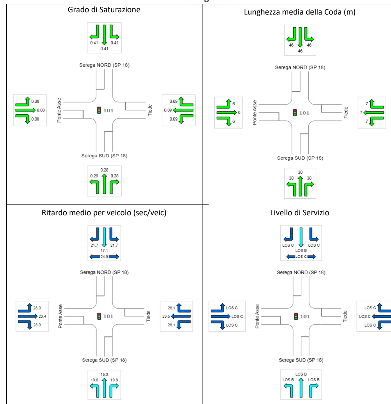
Figura 8-15: Nodo N04 – via Serega (SP 18) – via Ponte Asse – via Tiede Risultati delle verifiche di capacità - Ora di Punta 17.30-18.30 – SdP1
