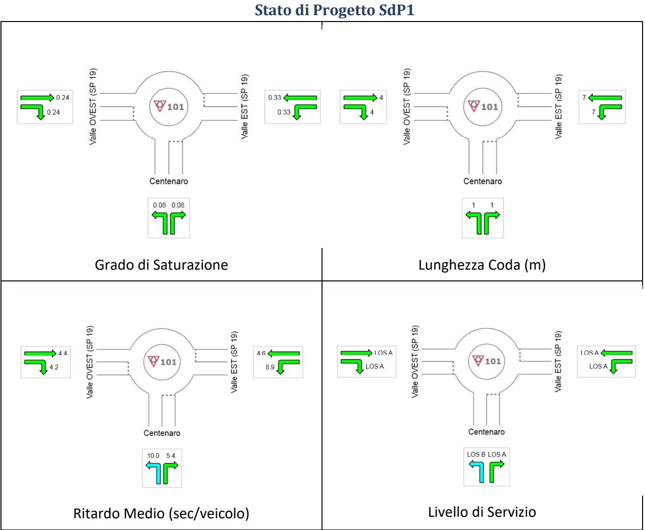
Figura 8-18: Nodo N05 – via Valle (SP 19) – via Centenaro Risultati delle verifiche di capacità - Ora di Punta 17.30-18.30 – SdP1
