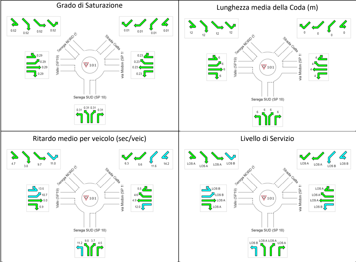
Figura 8-3: Nodo N01 via Serega (SP 18) – via Valle (SP 19) – via Modon (SP 19) – via Strada Gatta Risultati delle verifiche di capacità - Ora di Punta 17.30-18.30 – SdF
