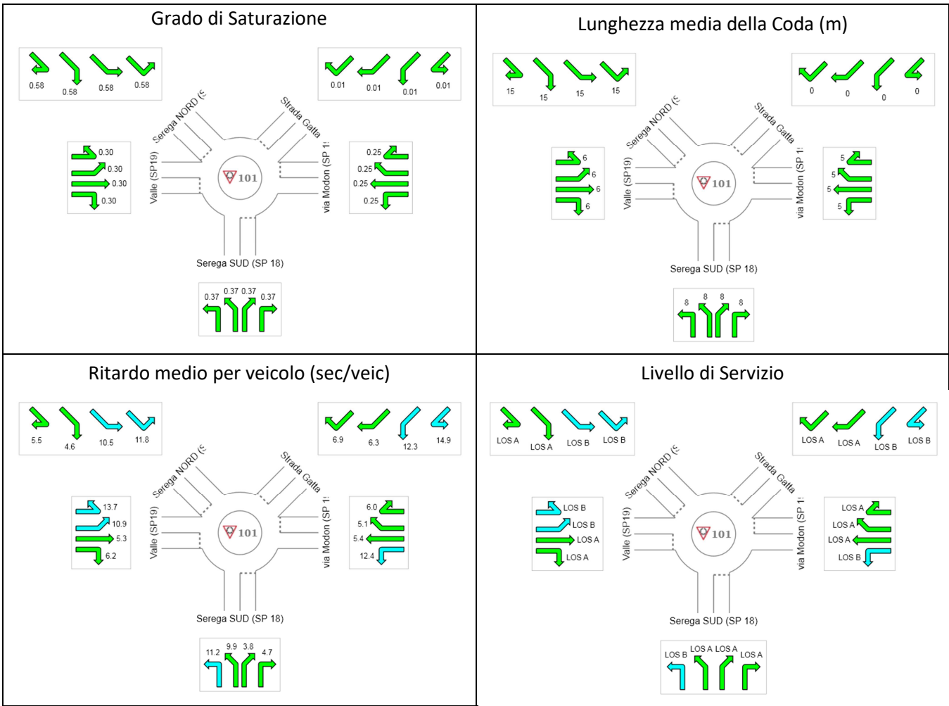
Figura 8-4: Nodo N01 via Serega (SP 18) – via Valle (SP 19) – via Modon (SP 19) – via Strada Gatta Risultati delle verifiche di capacità - Ora di Punta 17.30-18.30 – SdP1
