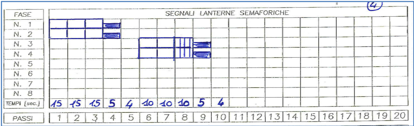
Figura 8-9: Fasatura dell’IS del nodo N03
