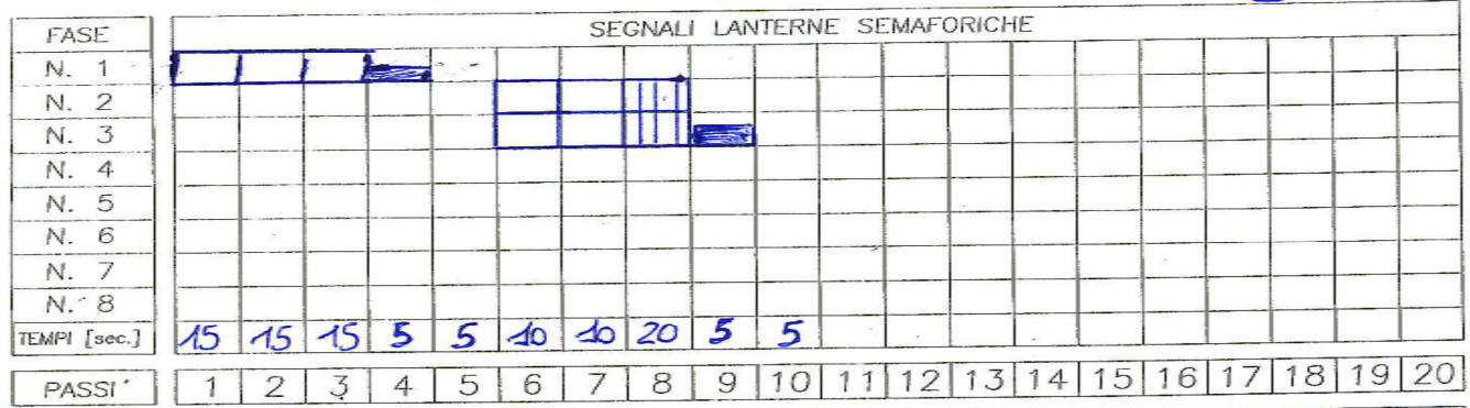
Figura 8-13: Fasatura dell'IS del nodo N04
