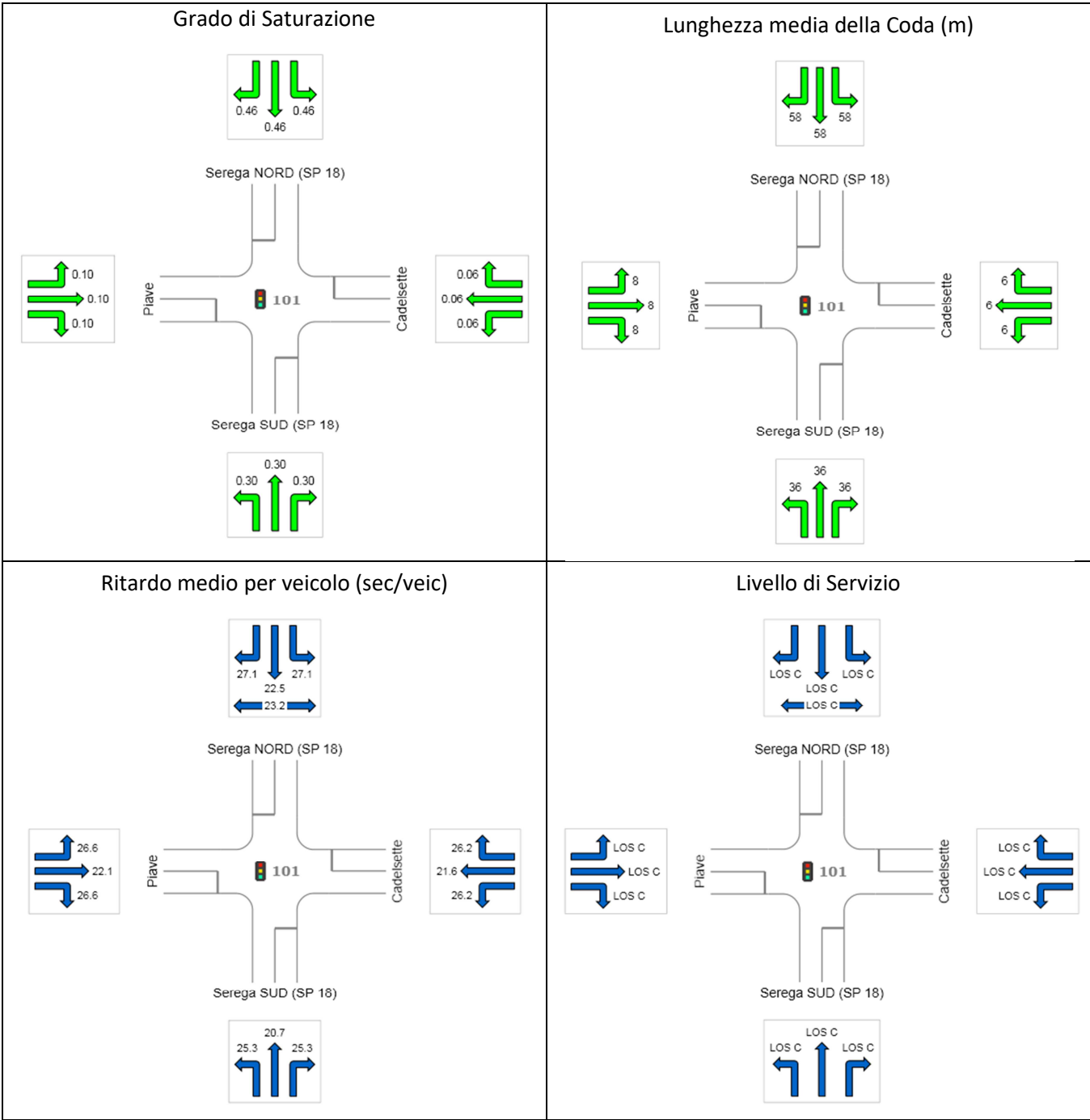
Figura 8-11: Nodo N03 – via Serega (SP 18) – via Cadelsette – via Piave Risultati delle verifiche di capacità - Ora di Punta 17.30-18.30 – SdP1
