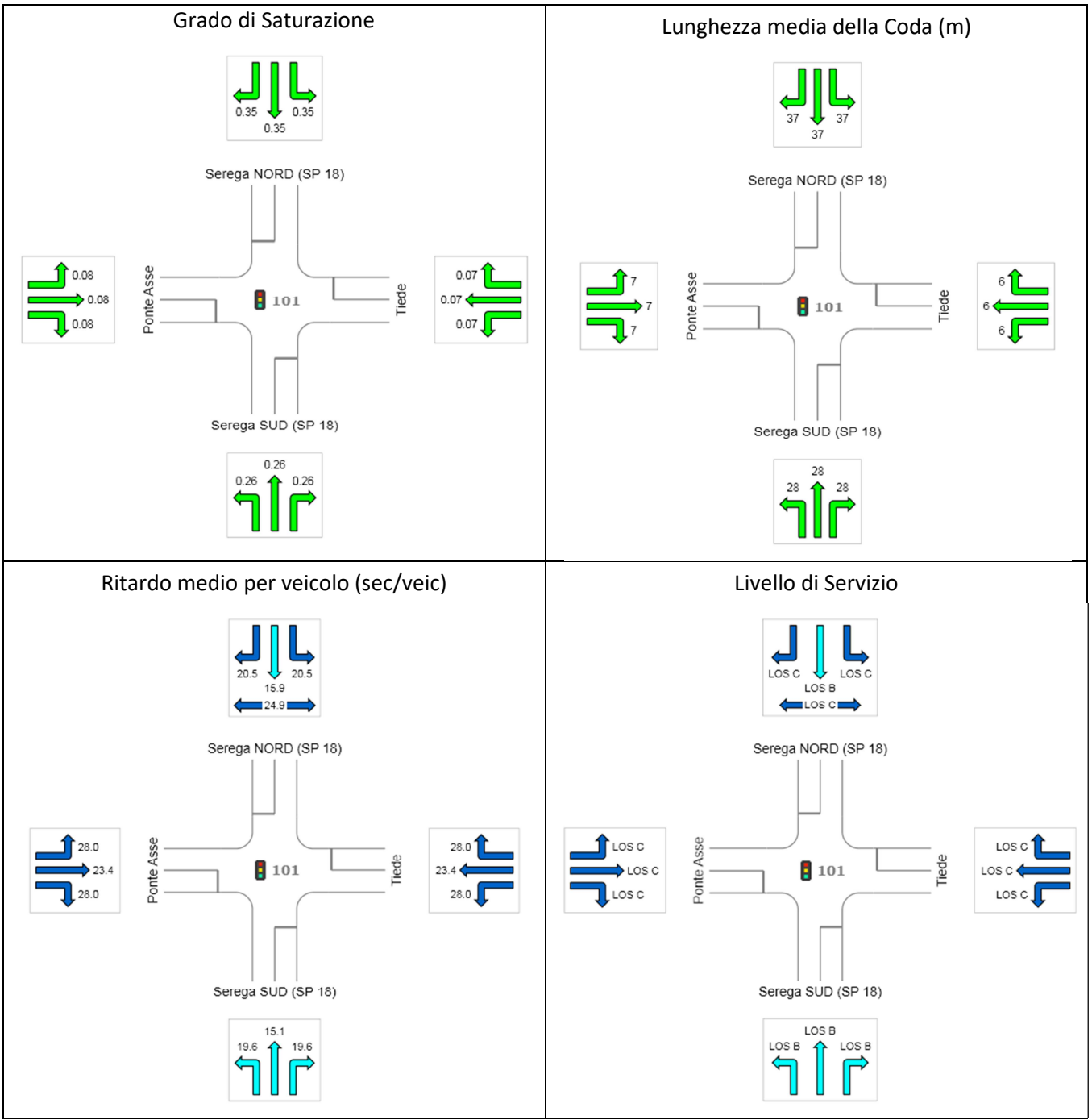
Figura 8-14: Nodo N04 – via Serega (SP 18) – via Ponte Asse – via Tiede Risultati delle verifiche di capacità - Ora di Punta 17.30-18.30 – SdF
