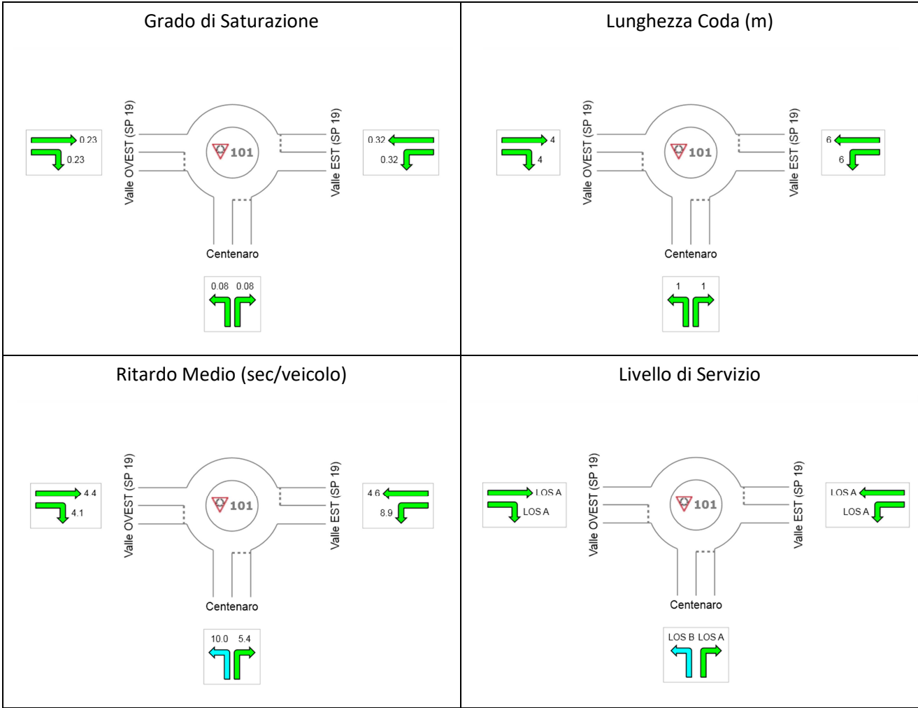
Figura 8-17: Nodo N05 – via Valle (SP 19) – via Centenaro Risultati delle verifiche di capacità - Ora di Punta 17.30-18.30 – SdF
