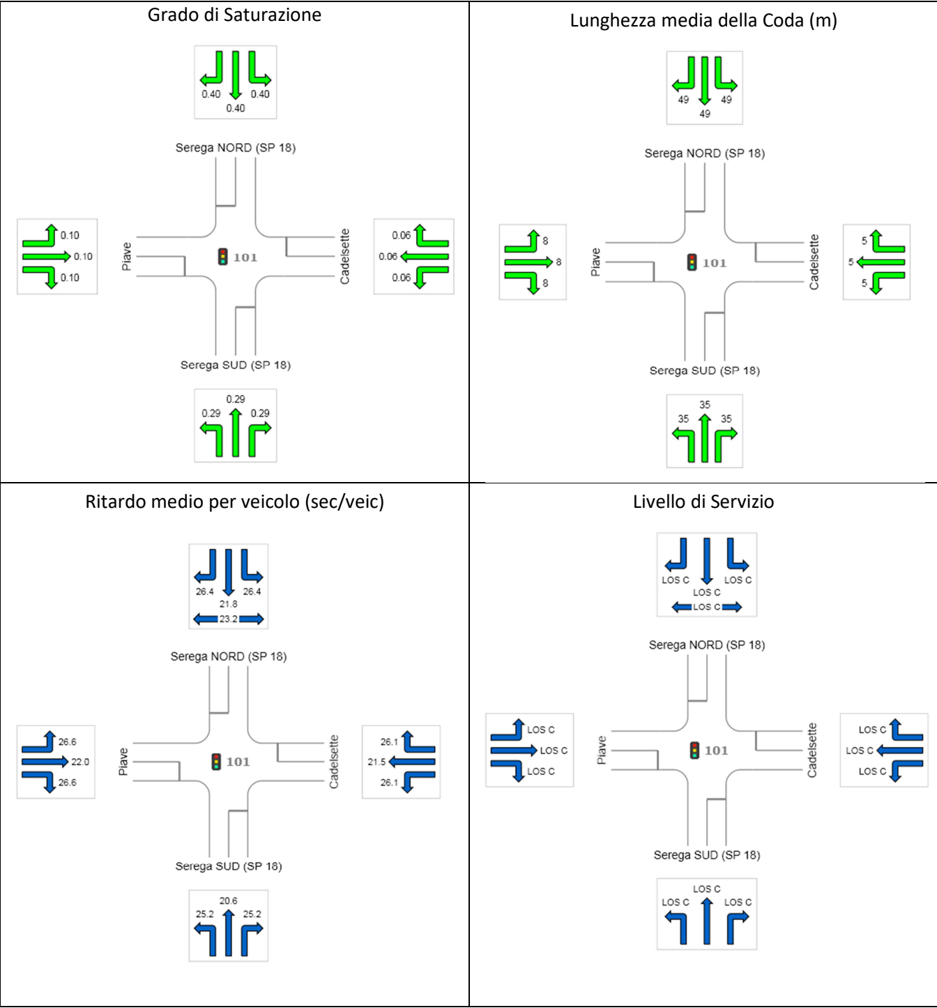
Figura 8-10: Nodo N03 – via Serega (SP 18) – via Cadelsette – via Piave Risultati delle verifiche di capacità - Ora di Punta 17.30-18.30 – SdF
