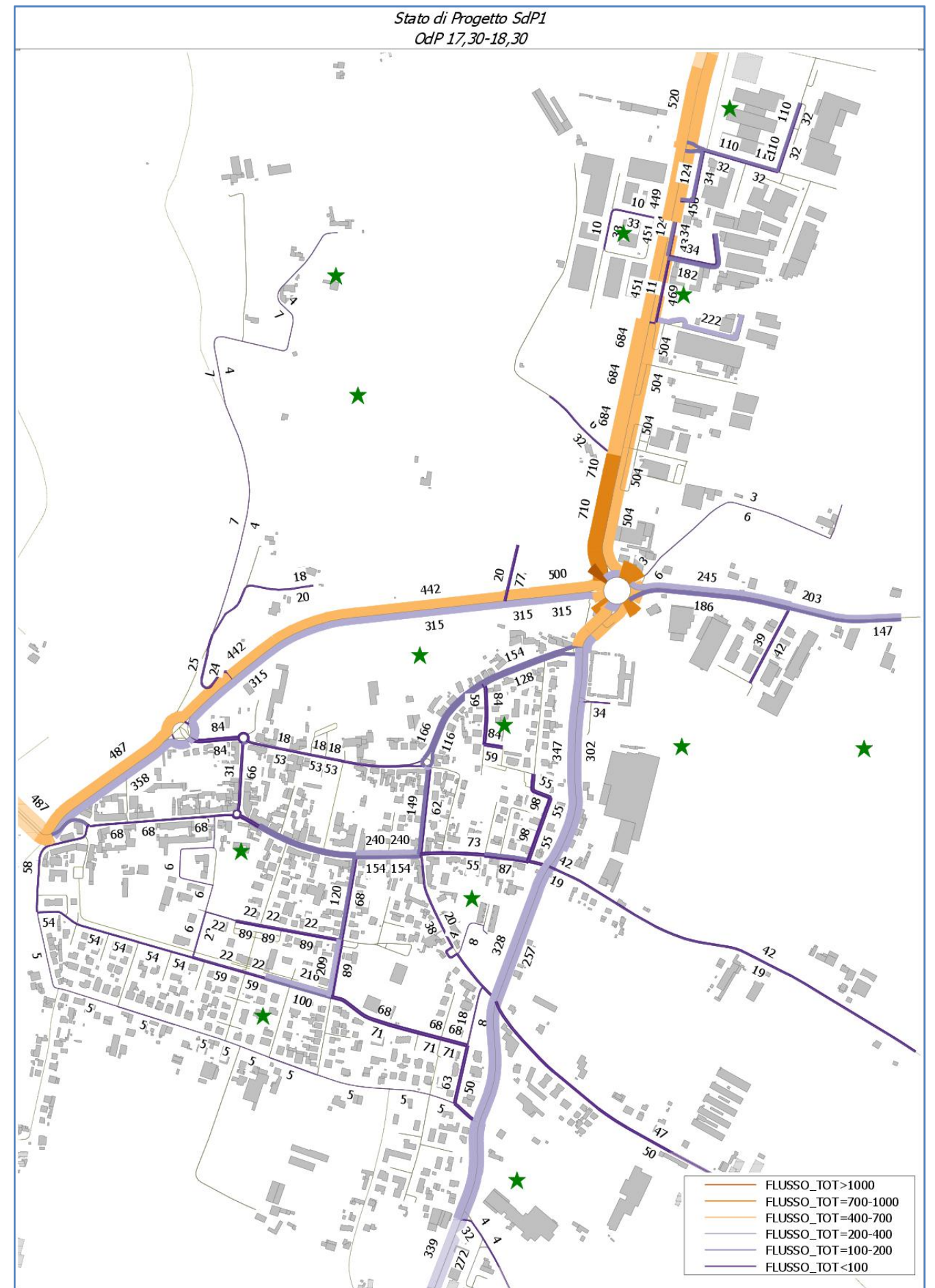
Figura 7-3: Flussogramma Ora di Punta 17.30-18.30 - Stato di Progetto SdP1
