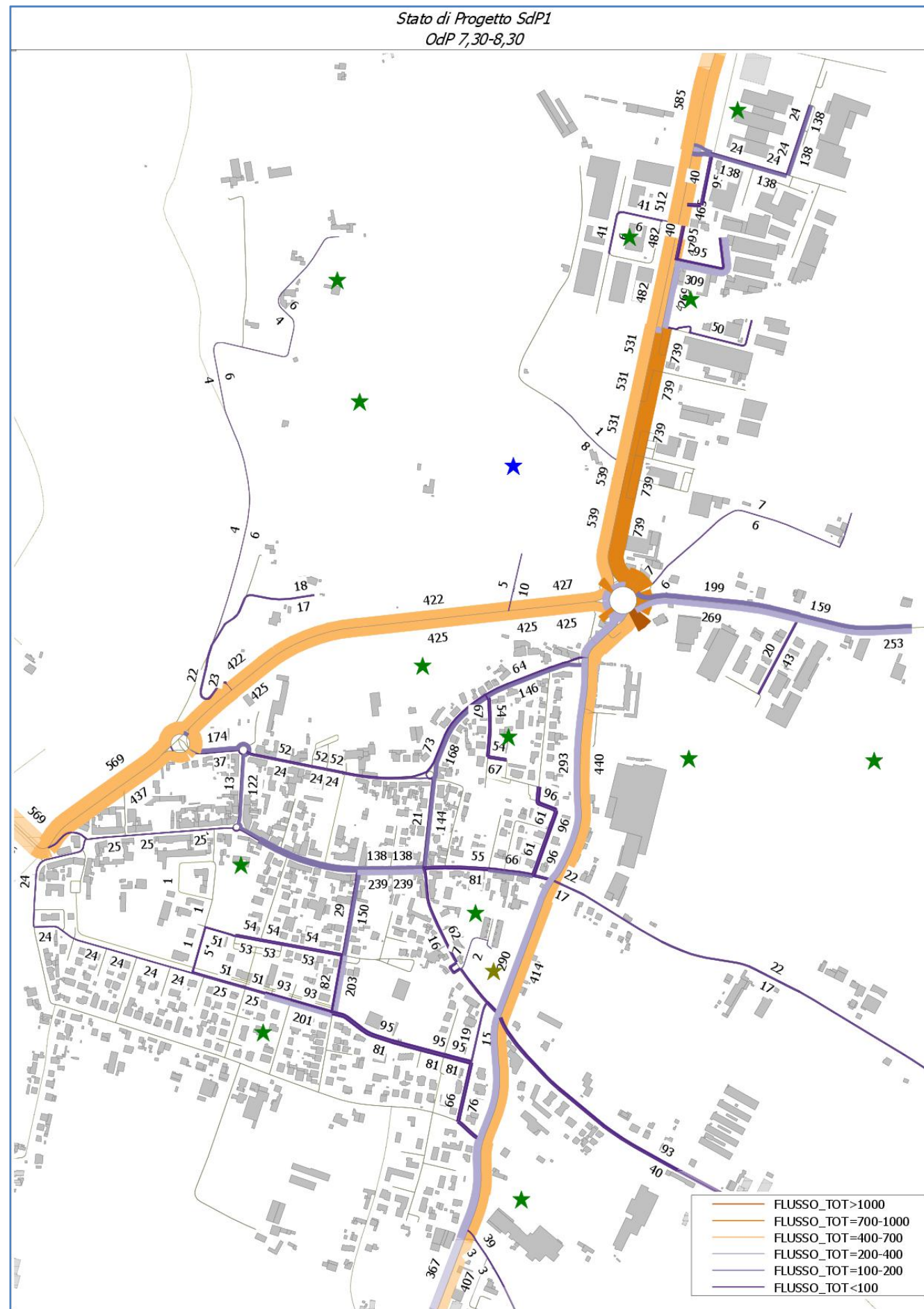
Figura 7-2: Flussogramma Ora di Punta 7.30-8.30 - Stato di Fatto SdP1
