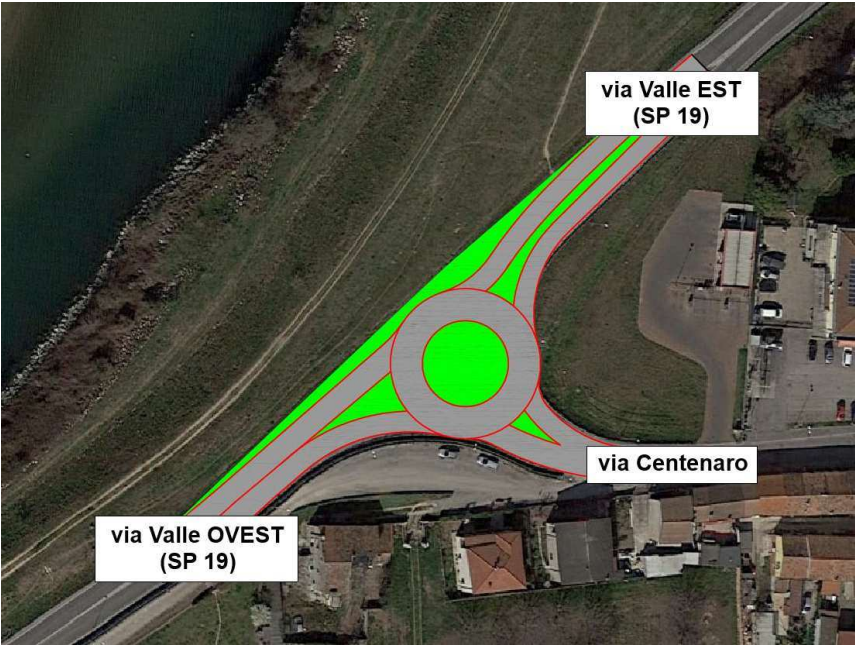
Figura 8-16: Nodo N05 – via Valle (SP 19) – via Centenaro Stato Attuale e di Progetto
