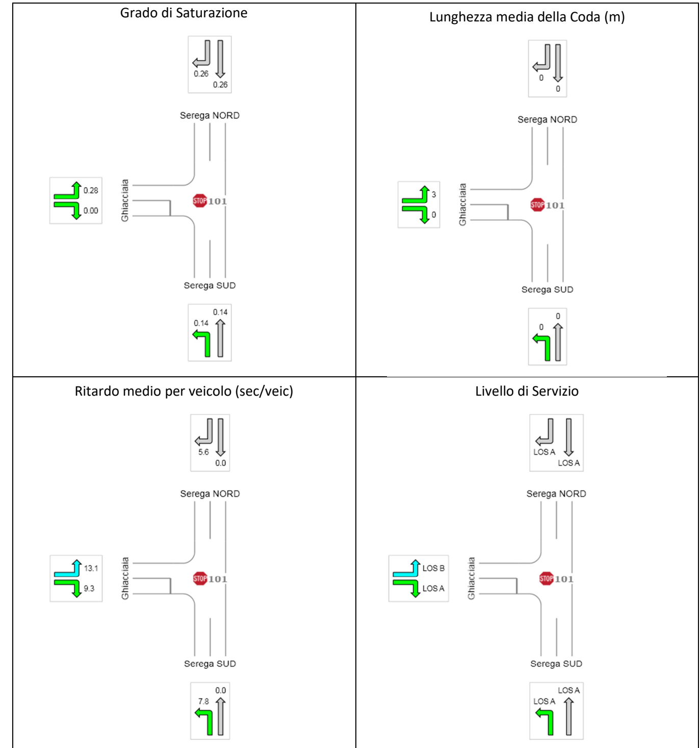
Figura 8-7: Nodo N02 – via Serega (SP 18) – via Ghiacciaia Risultati delle verifiche di capacità - Ora di Punta 17.30-18.30 – SdP1
