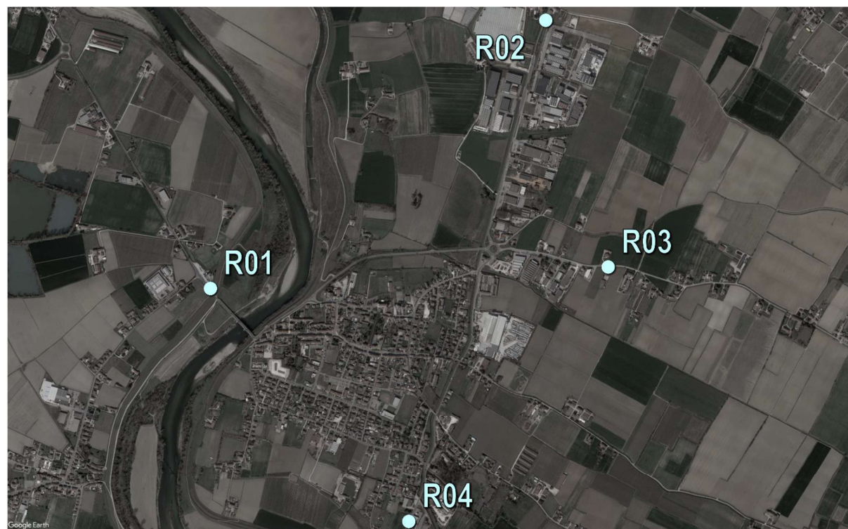
Figura 4-1: Ubicazione Rilievi di Traffico in continuo con radar
