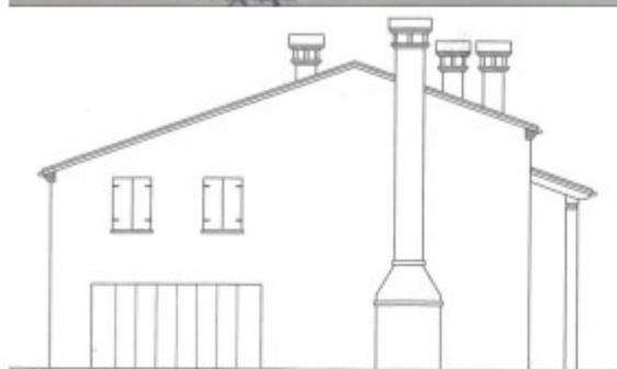
PROSPETTO OVEST
