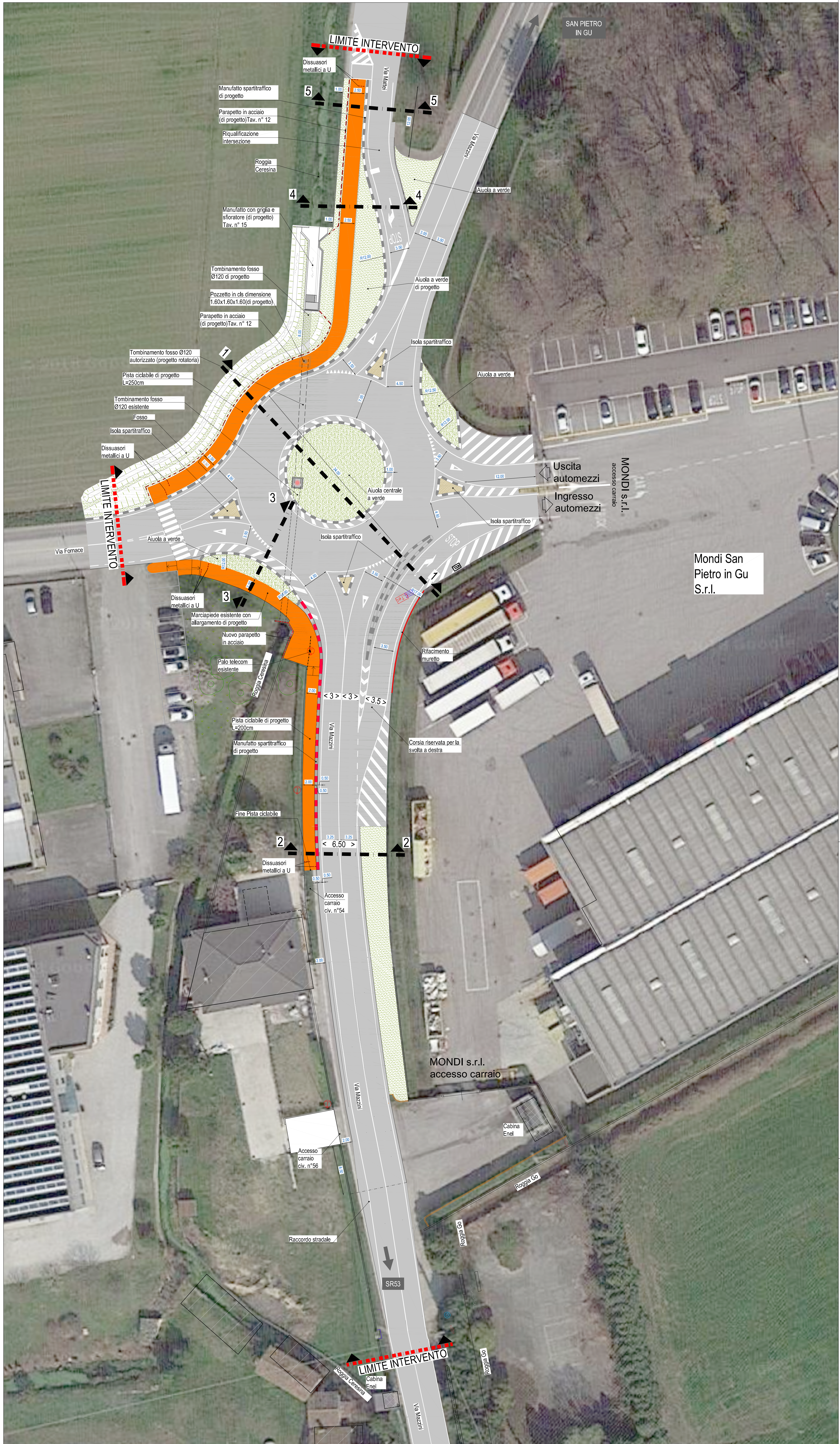
PLANIMETRIA DI PROGETTO scala 1:250
